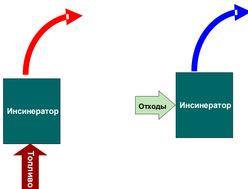
Рисунок 2-1 Технологическая схема для категории источников 5.С.2 Открытое сжигание отходов: левый столбик показывает процесс, когда энергия, образуемая при сжигании, восстанавливается (отходы используются в качестве топлива); правый столбик показывает ситуацию, когда энергия не восстанавливается
